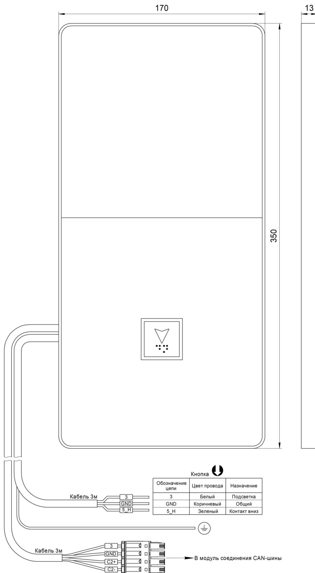
Рис.1 Внешний вид, габаритные и установочные размеры Вызывного поста МАЛАХИТ НШЕК.468381.089
